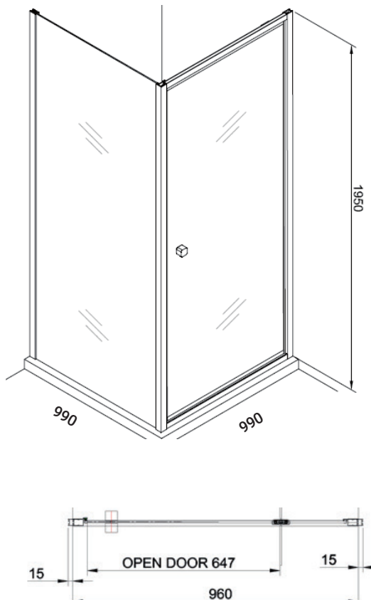
Shower Door
